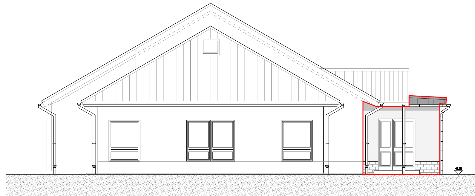
Ostansicht
